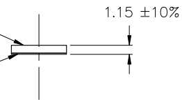
DETAIL 2 : 1
